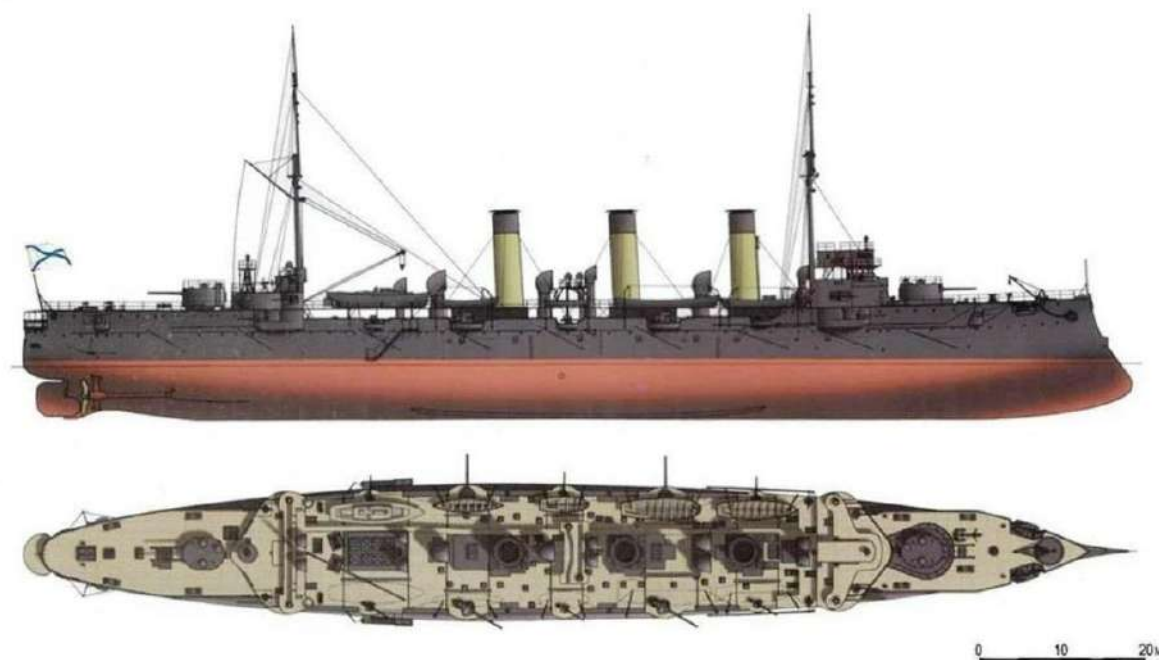
Рис. 3. Крейсер «Кагул»
