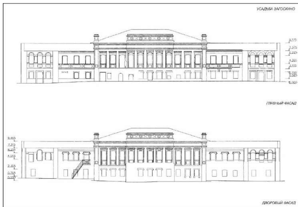
Рис. 6. Фасады усадьбы Загоскиных, с. Загоскино. Чертежи (Лапшина, 2019)
