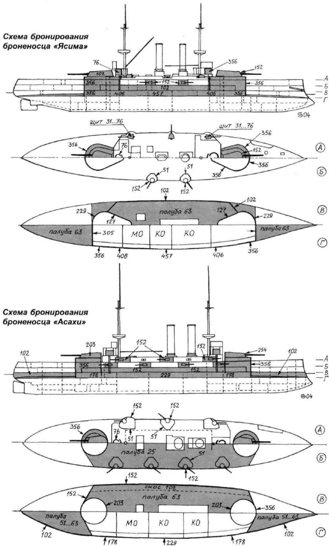
Рис. 4. Отличия в схеме бронирования судов типа «Фуджи»/«Яшима» от линкора «Асахи»
