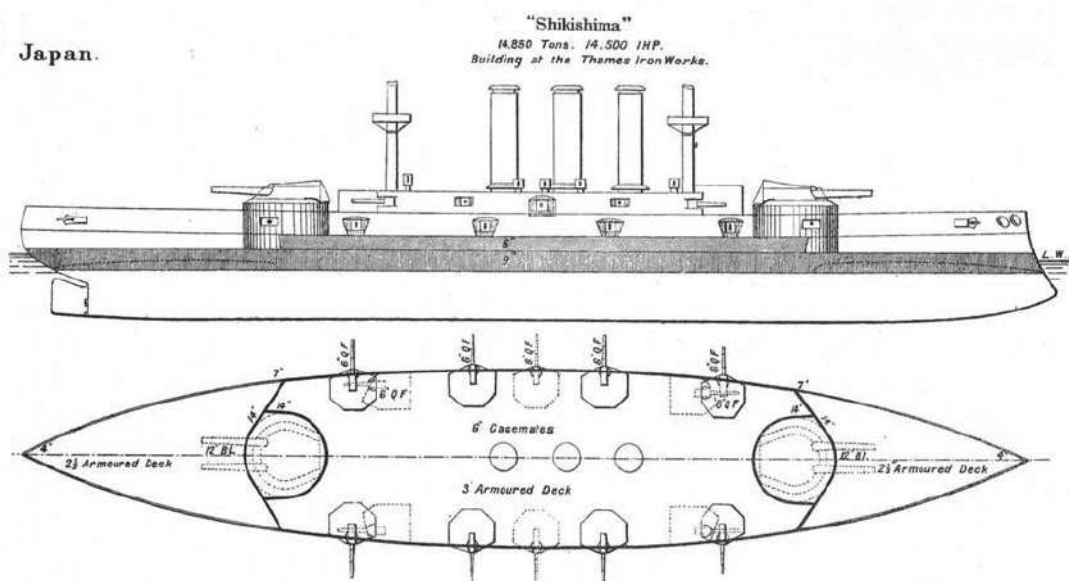
Рис. 6. Схема бронирования эскадренных броненосцев типа «Шикишима»
