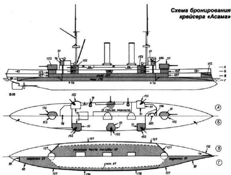
Рис. 6. Бронирование крейсеров типа «Асама» было, пожалуй, лучшим в мире в своем классе ко времени Русско-японской войны
