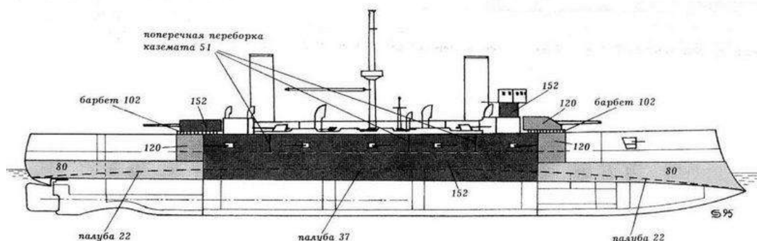
Рис. 8. Схема бронирования «Касуги» наглядно демонстрирует непревзойденную для крейсера площадь защиты корабля
