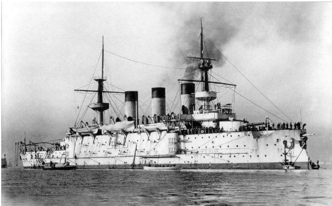
Рис. 9. «Броненосец-крейсер» «Пересвет» (1898) – русское оружие против перспективных японских броненосных крейсеров типа «Асама»: мореходный, но слабо бронированный и вооруженный, он больше предназначался для уничтожения тяжелых крейсеров противника и наиболее рискованных рейдерских операций вблизи военно-морских баз противника, нежели «плотного» эскадренного боя
