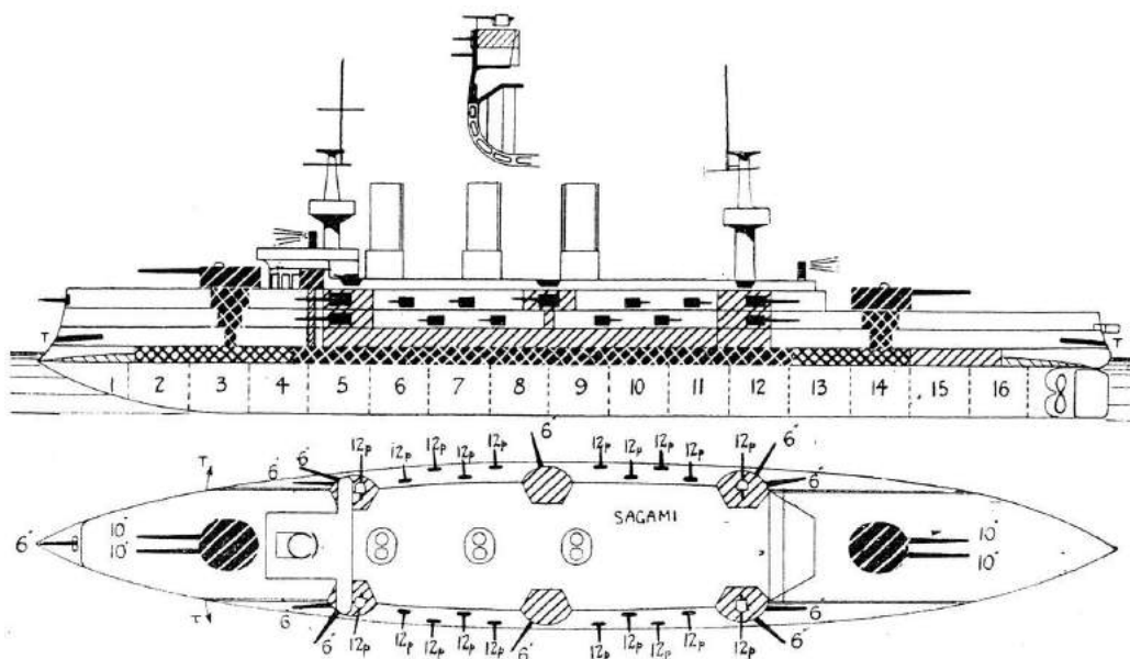
Рис. 10. Бронирование «Пересвета» было принесено в жертву крейсерским качествам (на схеме – захваченный японцами в Порт-Артуре и переименованный в «Сагами»)
