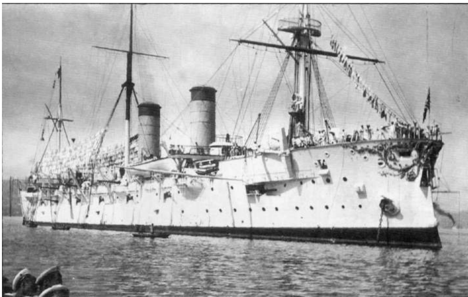
Рис. 3. Броненосный крейсер «Рюрик» (1892) – первое отечественное техническое воплощение полноценного бронированного рейдера
