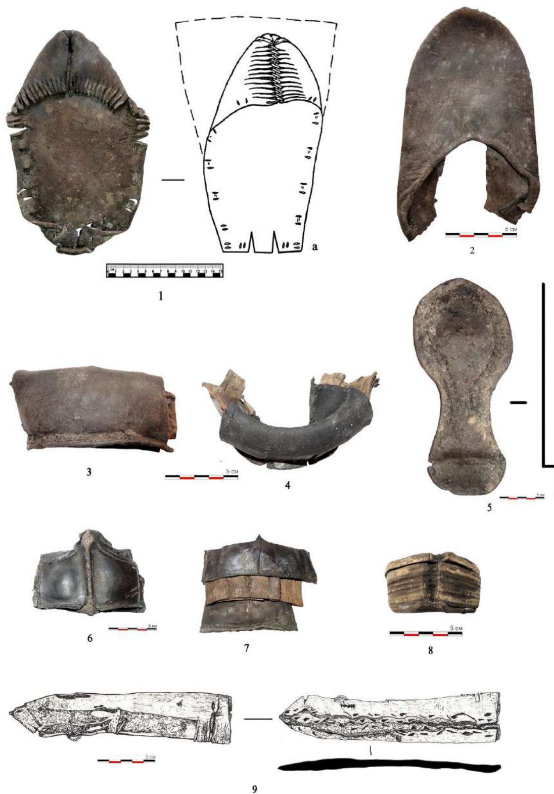
Рис. 1. 1 – простой поршень, а – форма края, 2 – головка туфли с цельнокроеным поднарядом, 3, 4 – жесткие задники моделей низкой обуви, 5 – подошва с крокулем, 6 – задник сапожный, 7 – детали жесткого задника, 8 – каблук наборный, 9 – ножны от короткого клинкового оружия (тесака)
