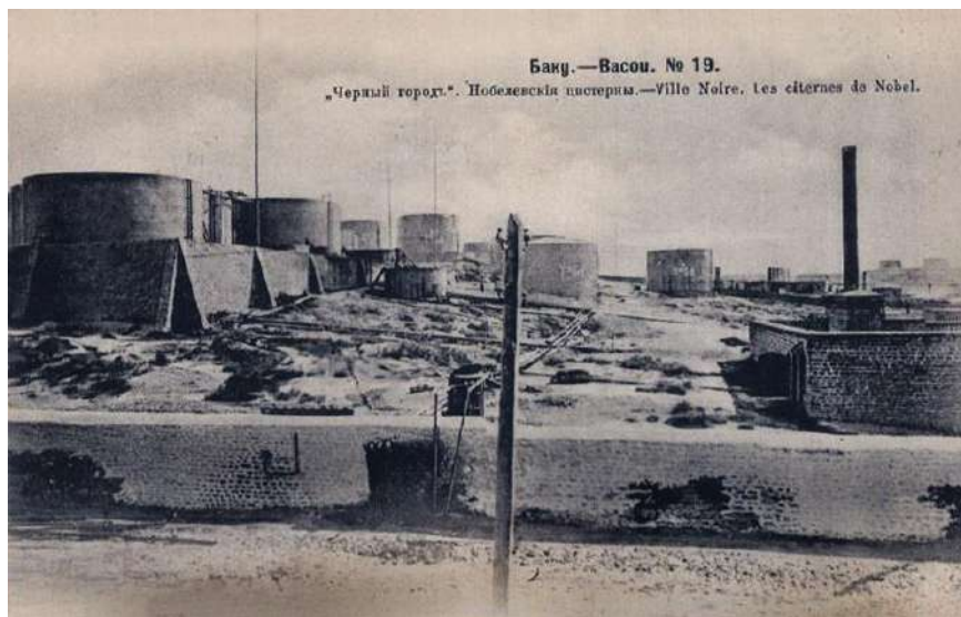
Рис. 4. Резервуары Шухова в Баку. До 1910 г.
