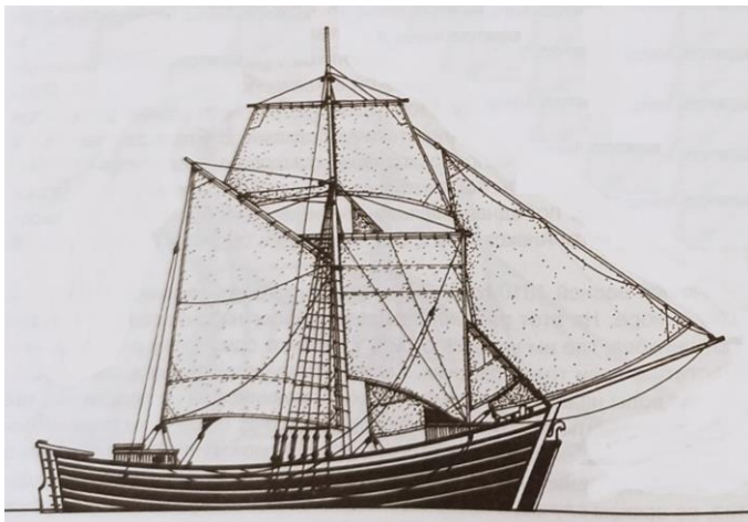
Рис. 1. Косовая (кусовая) лодка – каспийское рыболовное судно (Кирокосян, 2007: 150)
